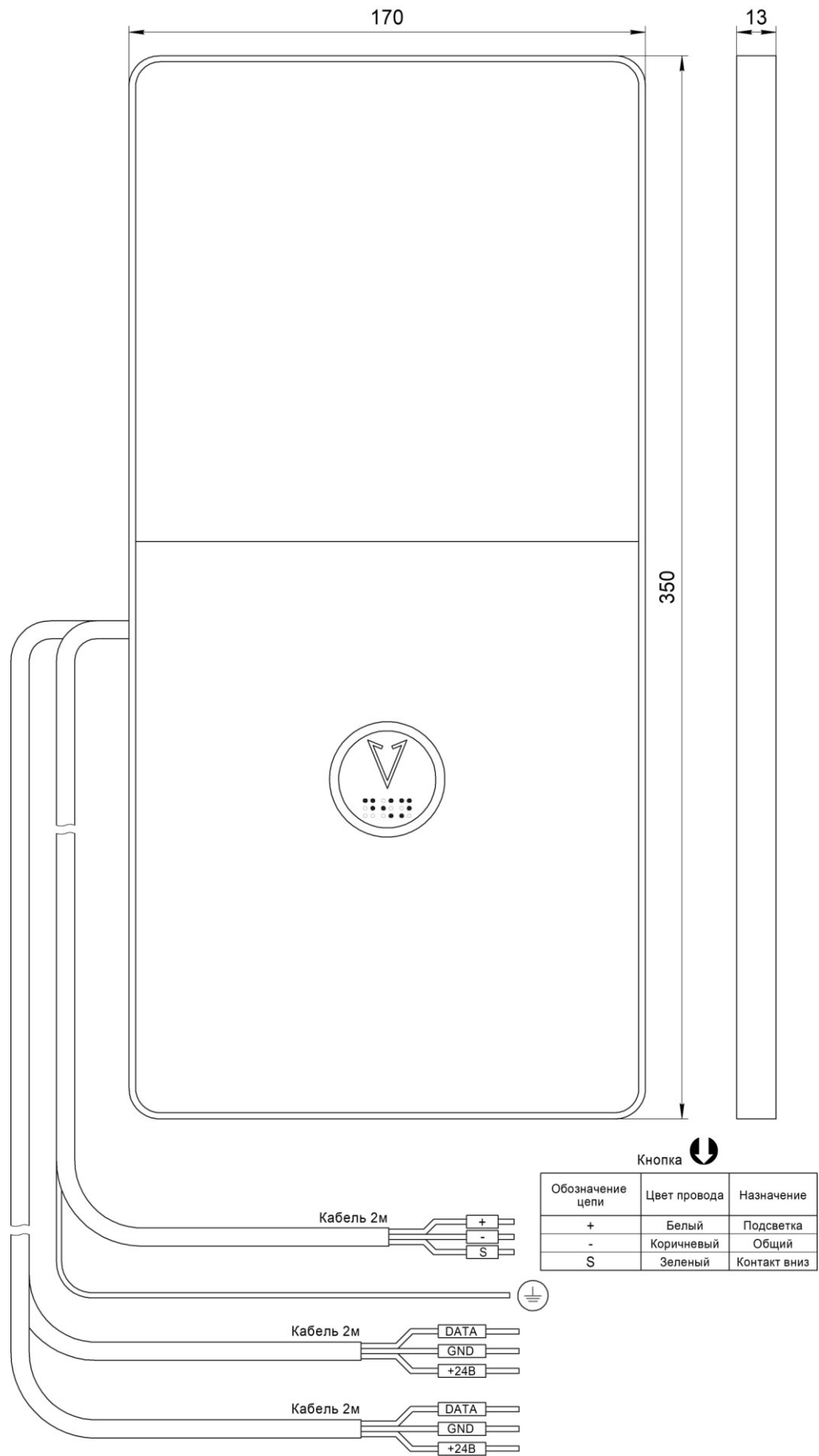
Рис.1 Внешний вид, габаритные и установочные размеры Вызывного поста GOLD НШЕК.468381.202-01
